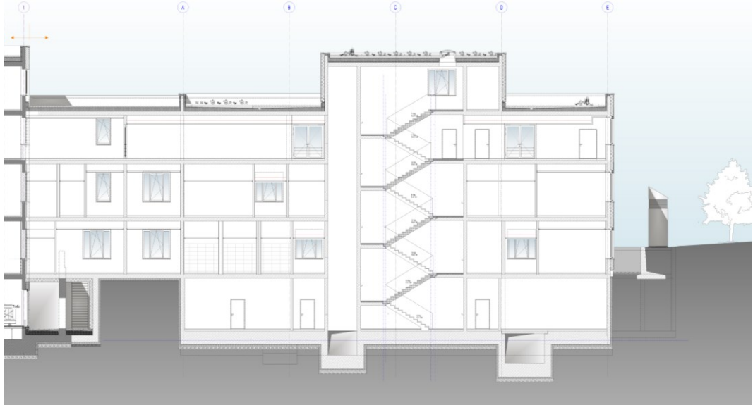
SCHNITT A-A
