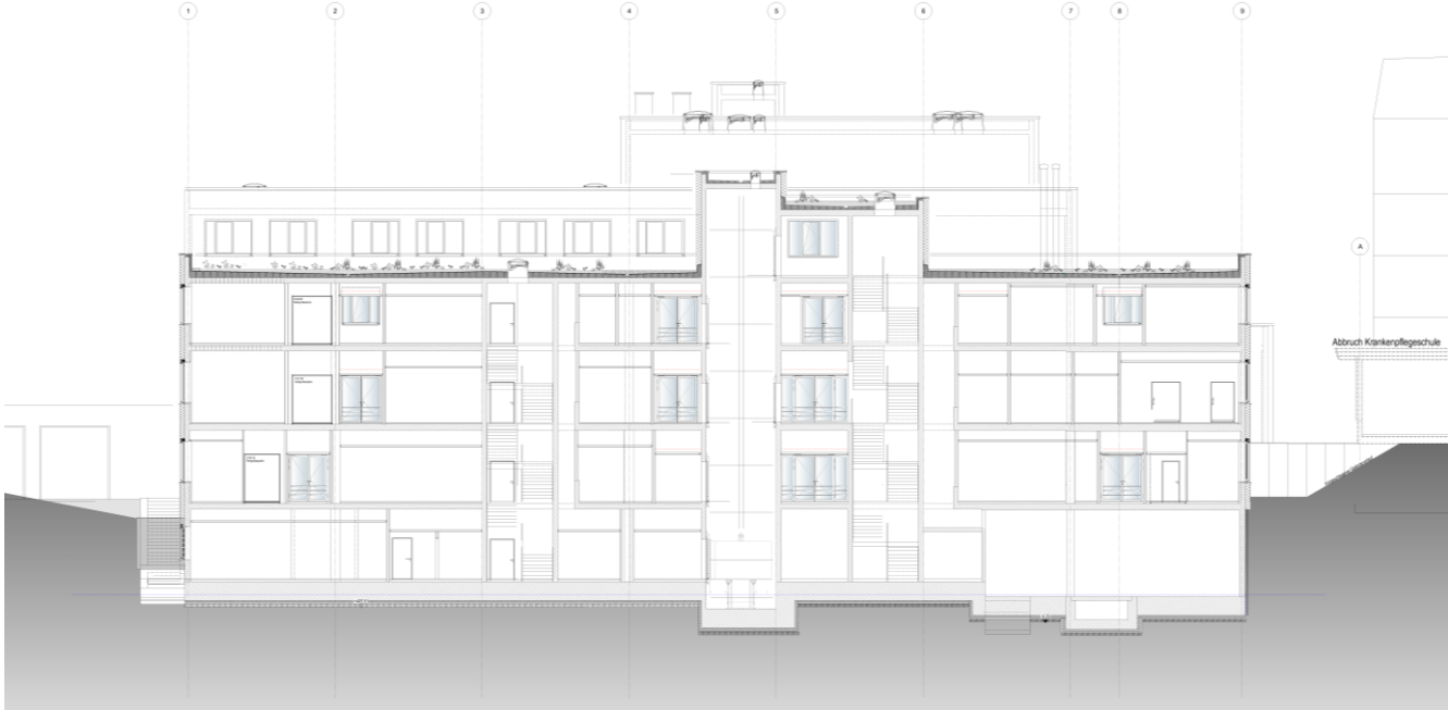
SCHNITT B-B
