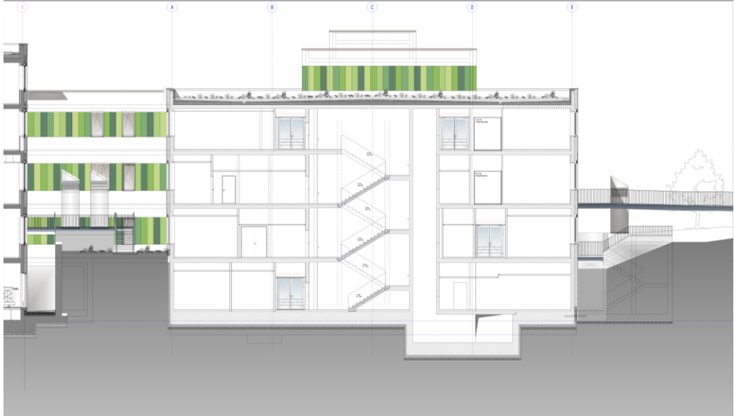
SCHNITT D-D
