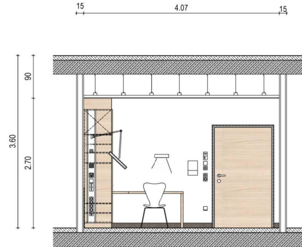
Wandansicht B
