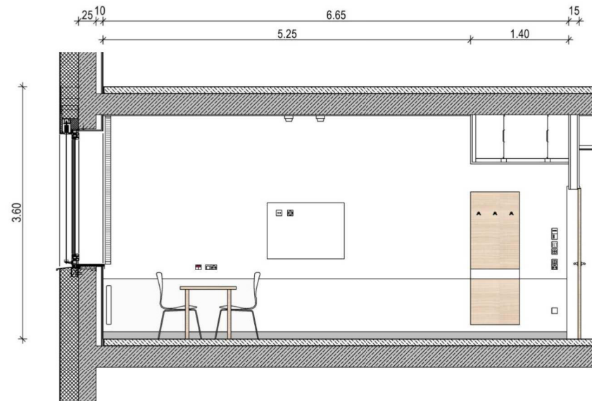
Wandansicht D
