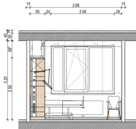
Wandansicht A
