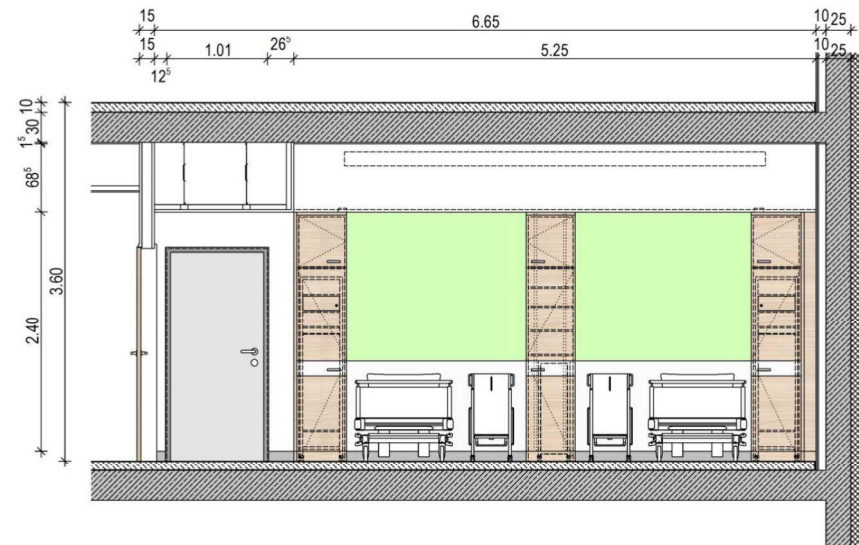
Wandansicht D
