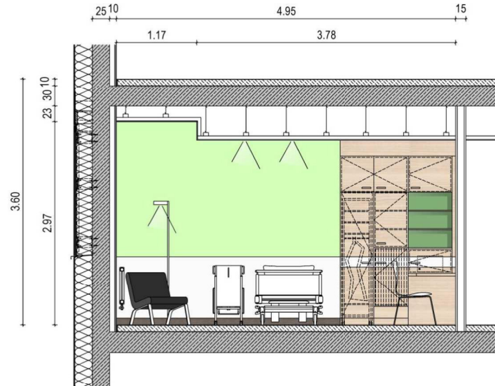
Wandansicht A
