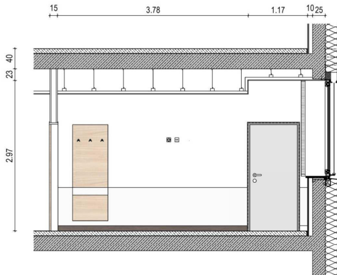
Wandansicht C
