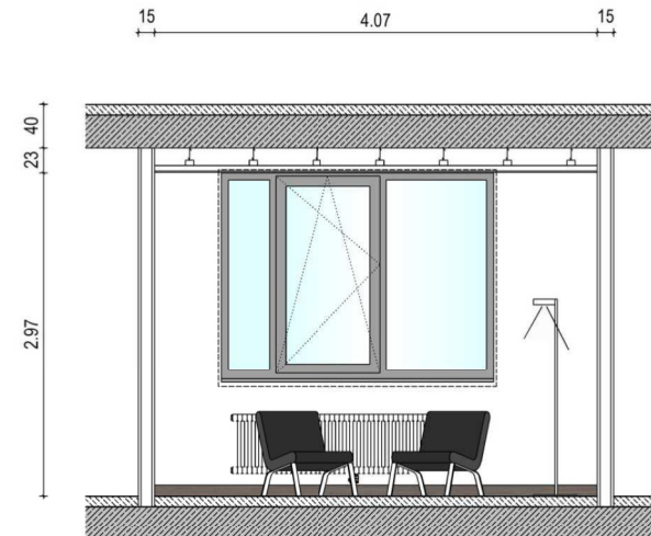
Wandansicht D
