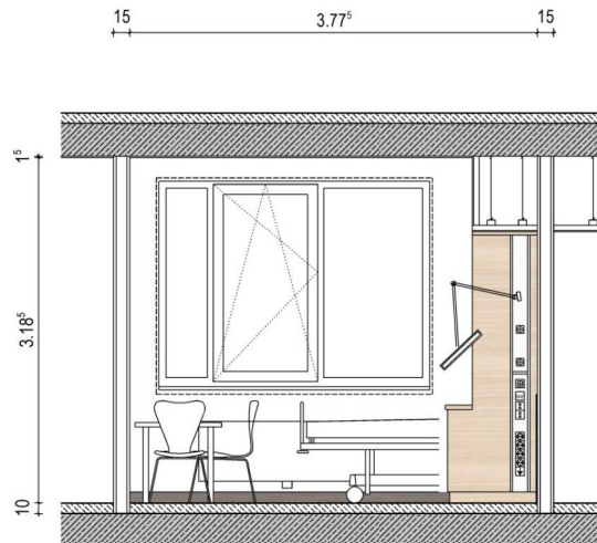
Wandansicht C
