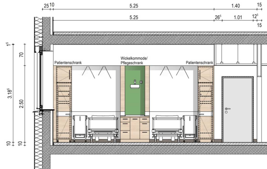
Wandansicht D
