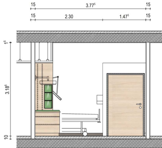
Wandansicht A
