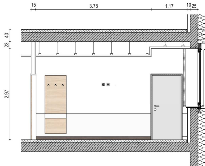
Wandansicht C
