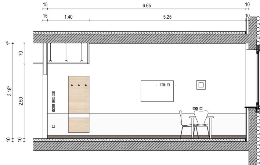
Wandansicht B
